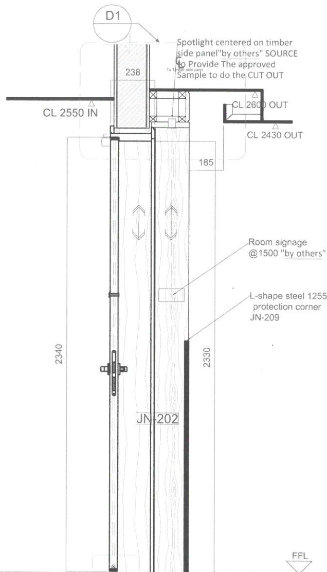
D2 SC1 Section
